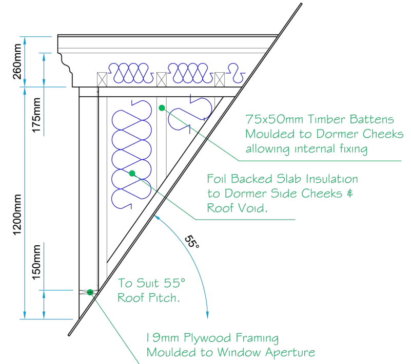
Section A-A
